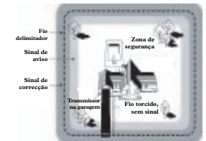
Zona de Segurança Maior Zona de Aviso Mais Pequena
